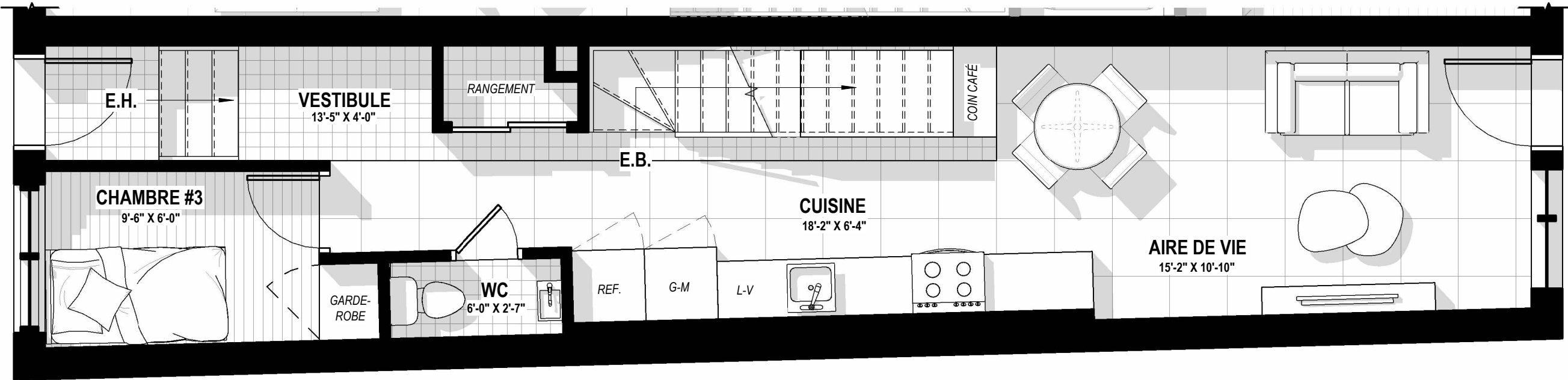
NIVEAU REZ-DE-CHAUSSÉE
