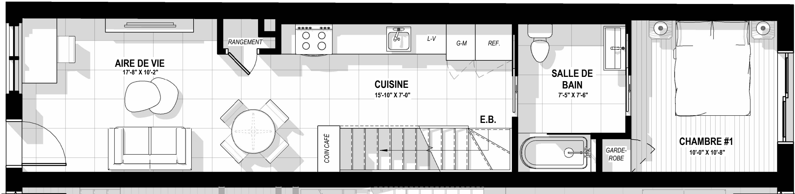
NIVEAU REZ-DE-CHAUSSÉE
